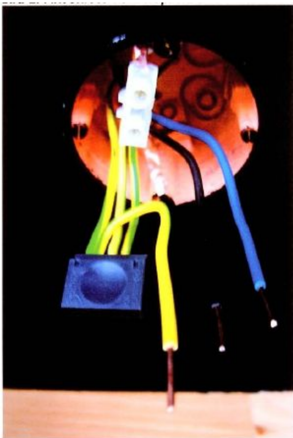
Рисунок 2: подключение медной ленты к электрической цепи розетки
