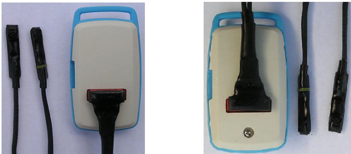
Рисунок 6. Способы подключения внешних микрофонов к диктфону ЛАБИ.423363.013 «СОРОКА-04».
