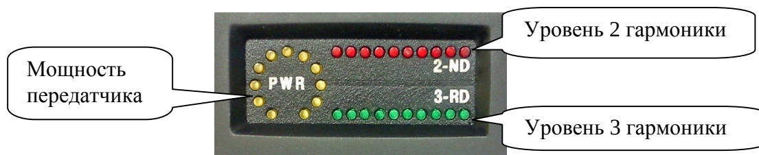
Рис. 3. Светодиодные индикаторы
